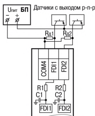
Рисунок 6.4 – Подключение к входам типа «ДС» датчиков с выходом р-п-р
