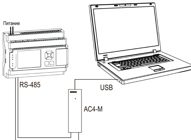
Рисунок 6.23 – Схема подключения прибора к ПК по RS-485
