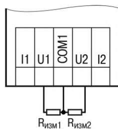
Рисунок 6.10 – Подключение резистивных датчиков
