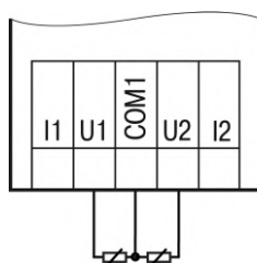
Рисунок 6.7 – Подключение ТС к аналоговому входу
