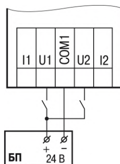
Рисунок 6.5 – Схема подключения к универсальным входам, работающим в дискретном режиме датчиков типа «сухой» контакт
