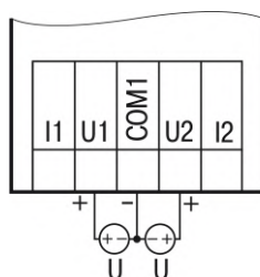
Рисунок 6.9 – Подключение датчиков с выходом в виде напряжения
