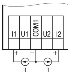
Рисунок 6.8 – Подключение датчиков с выходом в виде тока
