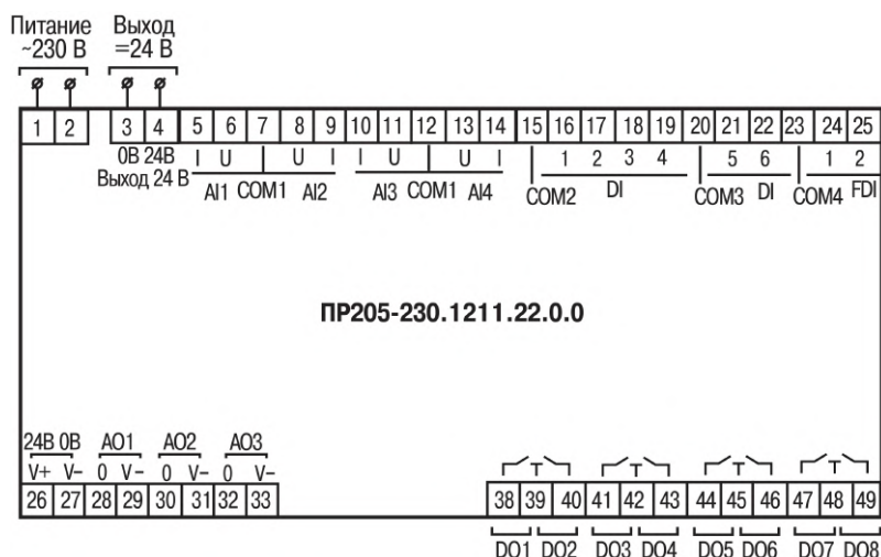
Рисунок А.1 – Расположение контактов для PR205-230.1211.22.0.0
