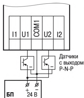
Рисунок 6.6 – Схема подключения к универсальным входам, работающим в дискретном режиме трехпроводных дискретных датчиков, имеющих выходной транзистор р-п-р-типа с открытым коллектором
