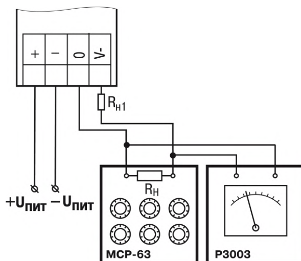
Рисунок В.3 – Схема подключения к ВЭ для юстировки сигналов типа «4...20 мА» ( R_H < 300 Ом)
