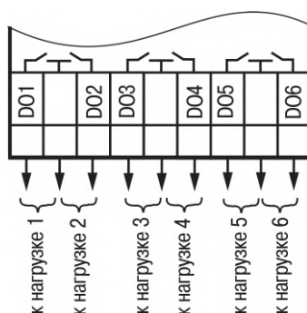
Рисунок 6.12 – Схема подключения ВЭ типа «Р»
