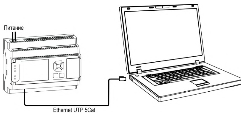
Рисунок 6.22 – Схема подключения прибора к ПК по Ethernet
