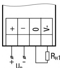
Рисунок 6.13 – Подключение аналогового выхода, находящегося в режиме источника тока
