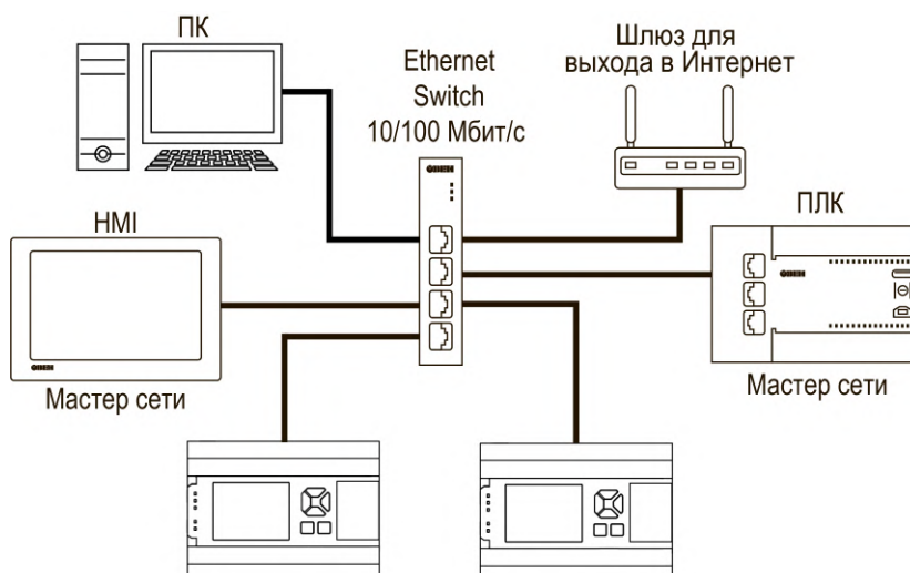
Рисунок 6.19 – Подключение по схеме «Звезда»
