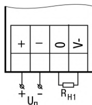
Рисунок 6.14 – Подключение аналогового выхода, находящегося в режиме источника напряжения
