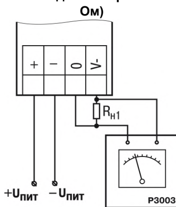
Рисунок В.4 – Схема подключения нагрузки к ВЭ для юстировки сигналов типа «0...10 В»
