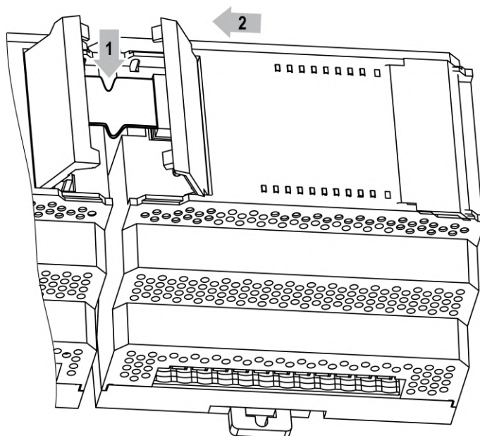
Рисунок 6.15 – Укладка шлейфа в углубление
