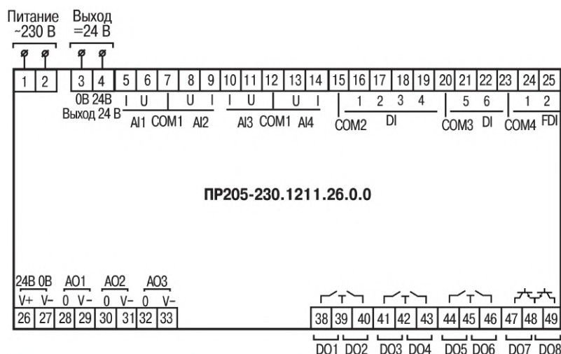
Рисунок А.3 – Расположение контактов для ПР205-230.1211.26.0.0
